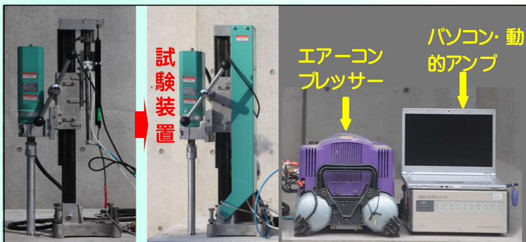
小口径コア型コンクリート強度診断試験機 (特許)
